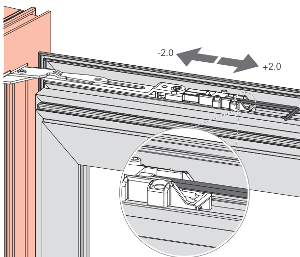
Fig. 10.1: Bisagra de compás de canal
