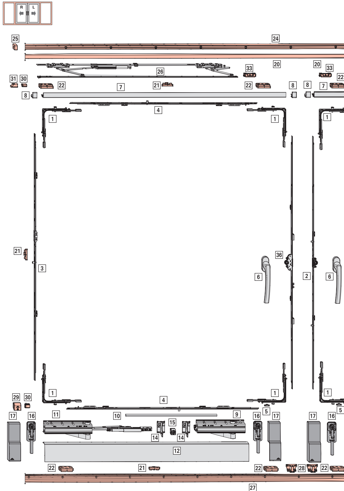
figura: hasta 160 kg; RC1 N; ancho canal de herraje [FFB] 1000; alto canal de herraje [FFH] 1300; cremona oscilobatiente cota variable; cremona oscilobatiente cota variable hoja pasiva sin cerradero soldado
