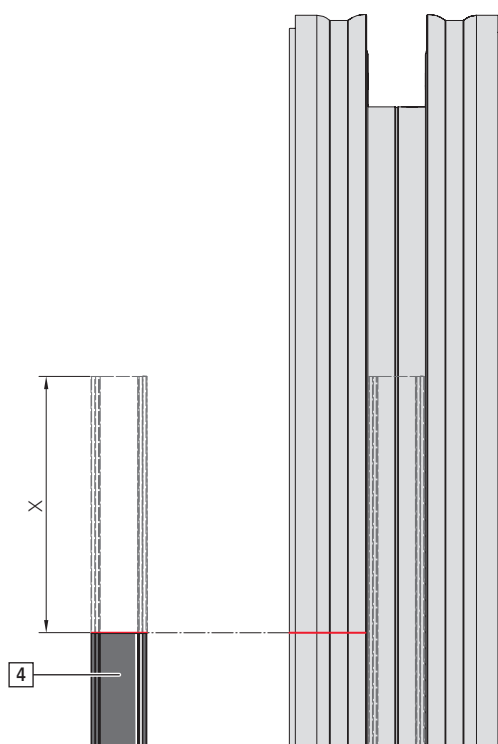
Fig. 10.1: La variante del prolongador de cremóna sin juego de deslizadores superiores en la hoja se muestra punteada.
