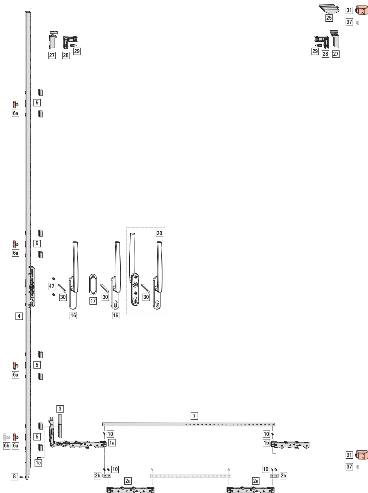
Fig. 4.2: imagen: diseño a la izquierda; AnH 1400 mm; AlH 2400 mm; PH 200 / 400 kg
