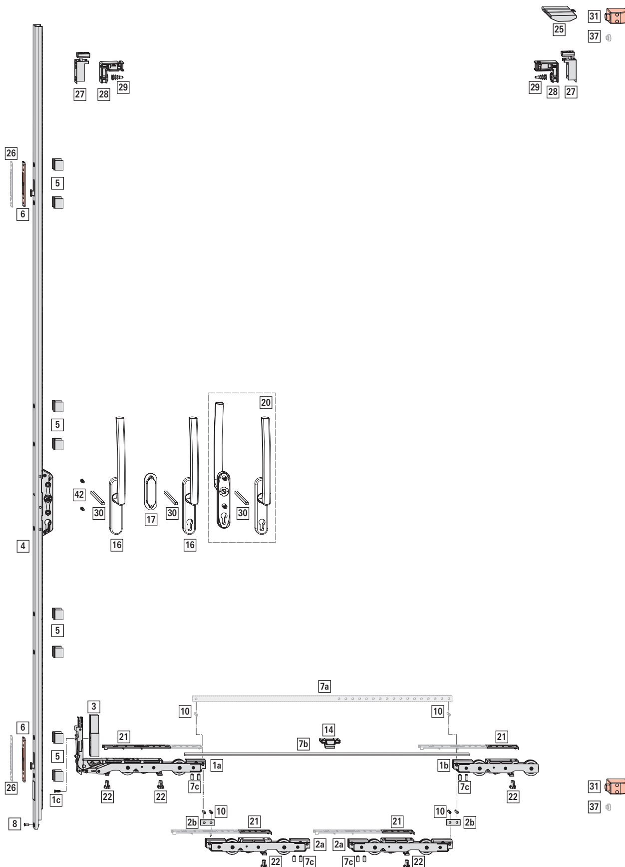
Fig. 4.5: imagen: diseño a la izquierda; AnH 1400 mm; AlH 2400 mm; PH 300 / 400 kg
