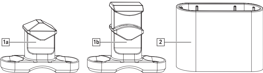
Fig. 8.1: [1a] bulón de cierre sin ventilación reducida; [1b] bulón de cierre con ventilación reducida; [2] suplemento
