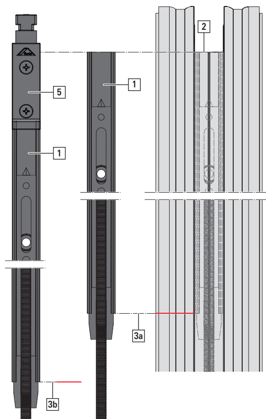
Fig. 10.1: La variante del prolongador de cremóna sin juego de deslizadores superiores en la hoja se muestra punteada.
